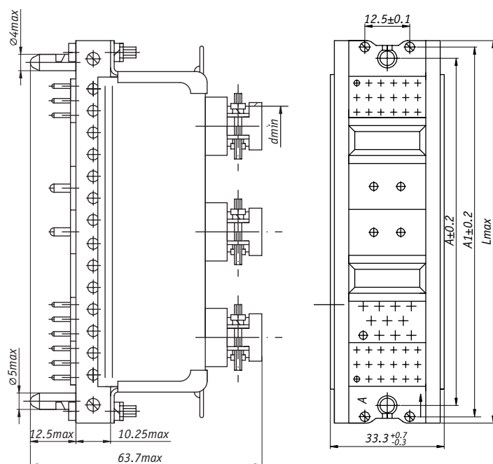
Рисунки 3 - Вилка приборно-кабельная с кожухом прямым
