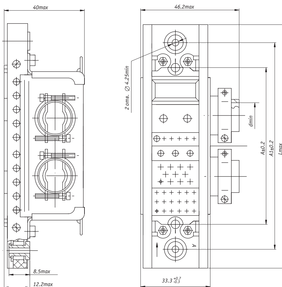
Рисунок 7 - Розетка блочная с кожухом угловым
