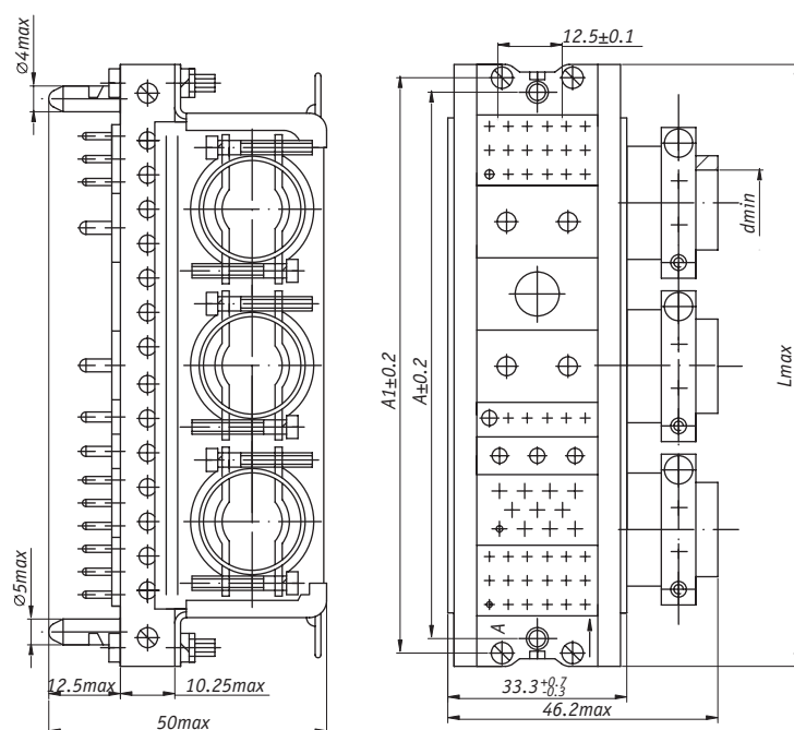
Рисунки 4 - Вилка приборно-кабельная с кожухом угловым
