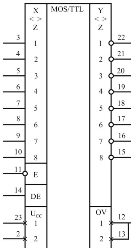
Рис. 1. Условное графическое обозначение микросхем 564ПУ9В, ОСМ564ПУ9В.
