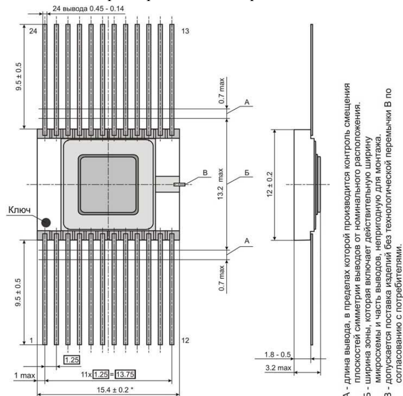
Рис.2. Корпус 4118.24-2.01 размеры в миллиметрах
