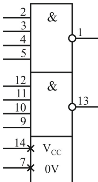
Рис. 1. Условное графическое обозначение микросхем 564ЛА8 ЭП.
