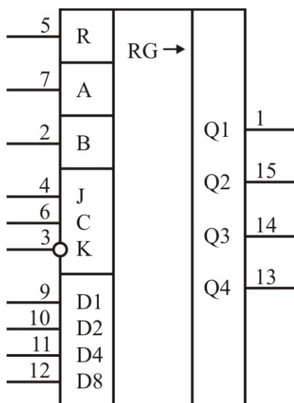
Рис. 1. Условное графическое обозначение микросхем 564ИР9В, Н564ИР9В, ОСМ564ИР9В.
