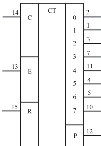
Рис. 1. Условное графическое обозначение микросхем 564ИЕ9В, Н564ИЕ9В, ОСМ564ИЕ9В.
